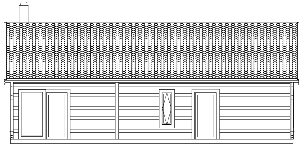
FASAD A1 1:100
