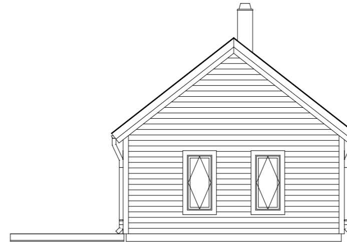
FASAD A2 1:100
