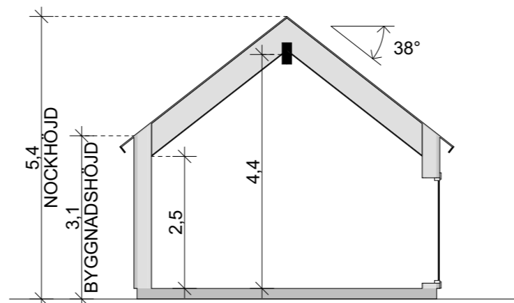
Sektion A2 1:100
