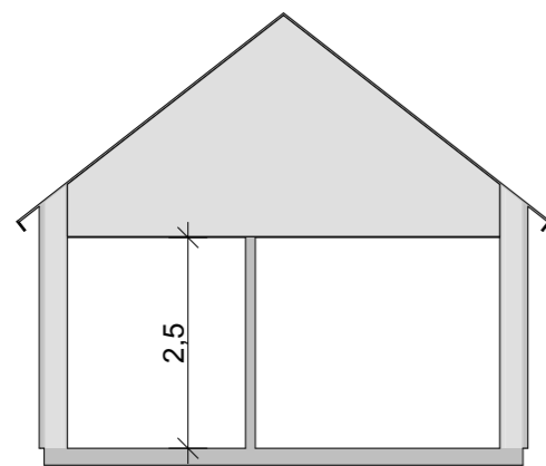
Sektion A1 1:100
