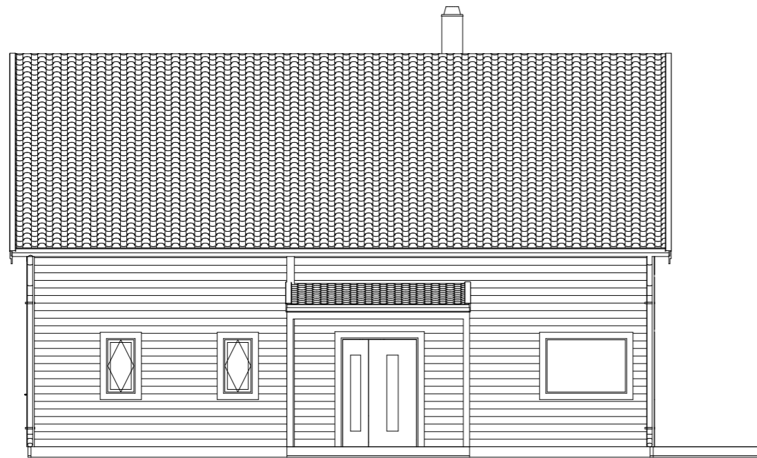
FASAD A3 1:100
