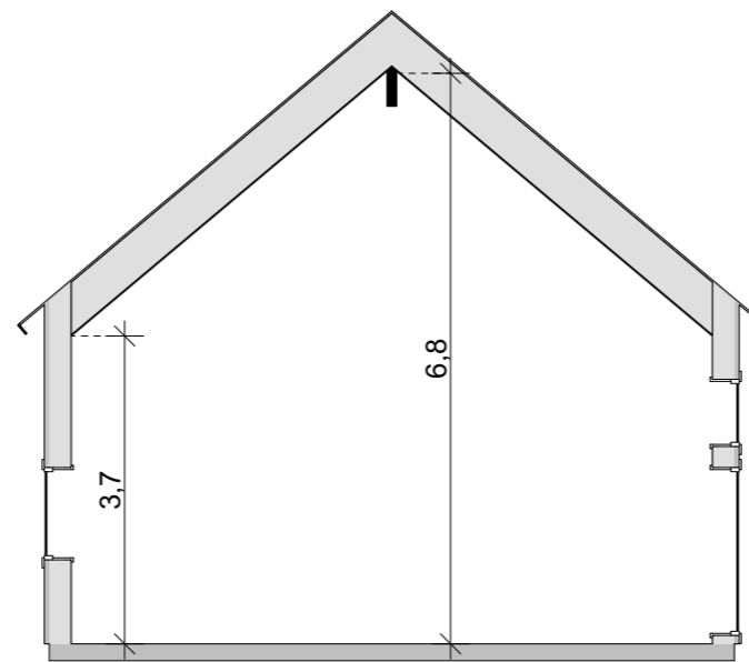
SEKTION A1 1:100
