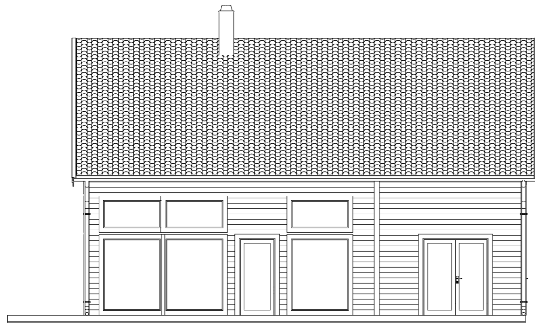
FASAD A1 1:100
