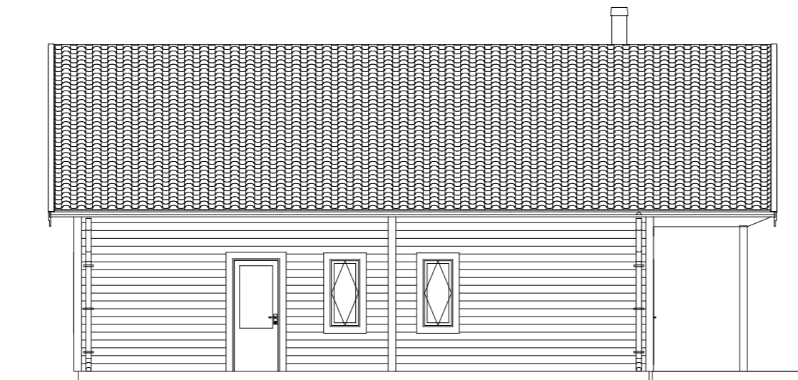
FASAD A1 1:100
