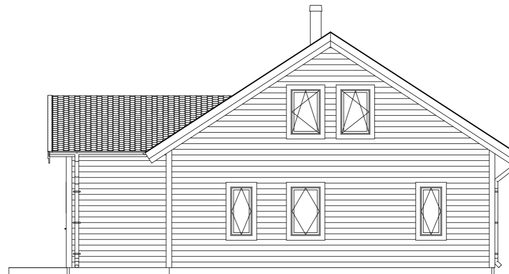
FASAD A4 1:100
