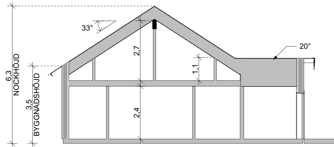
SEKTION A 1:100
