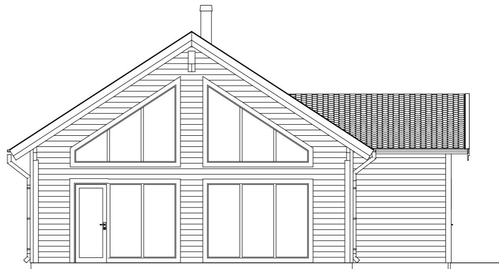
FASAD A2 1:100
