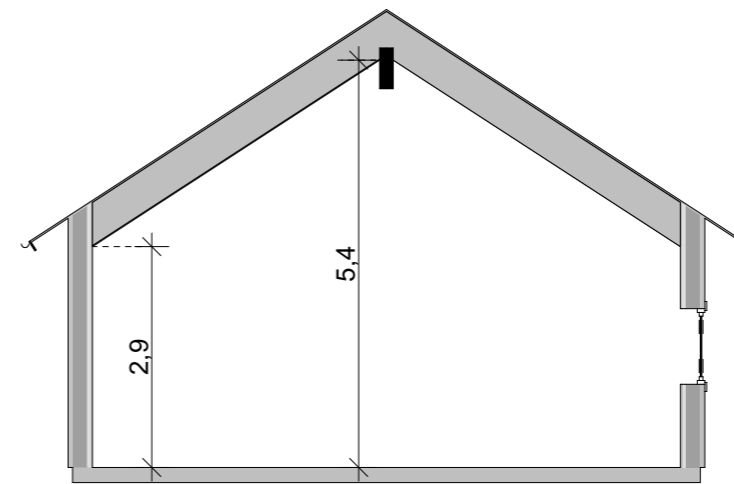
SEKTION B 1:100
