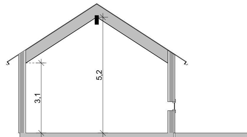
SEKTION B 1:100
