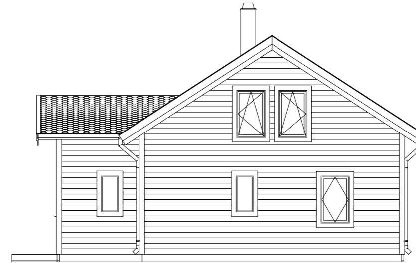
FASAD A4 1:100
