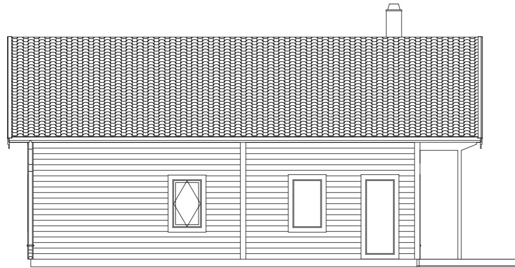
FASAD A1 1:100
