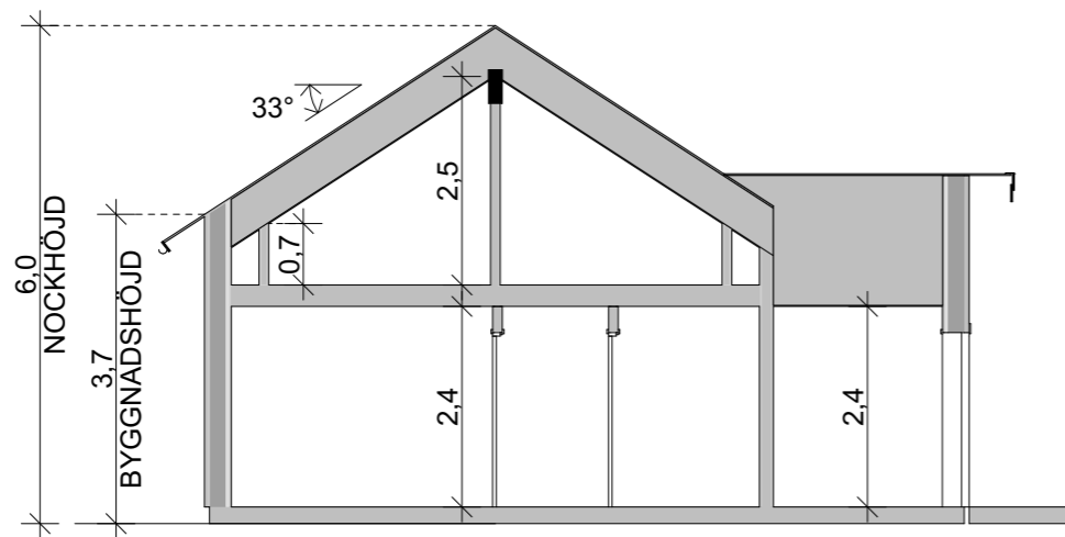
SEKTION A 1:100
