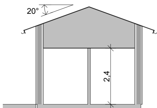
SEKTION C 1:100
