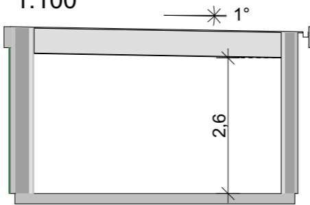
Sektion A2-A2 1:100
