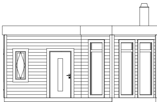
FASAD A2 1:100
