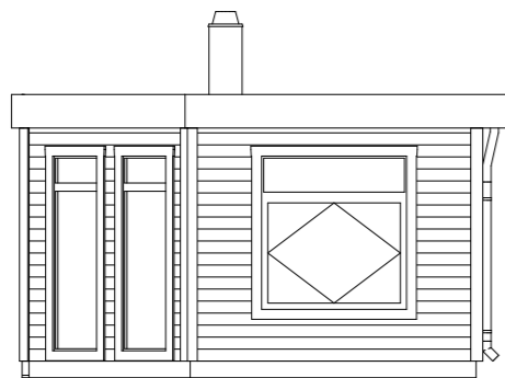
FASAD A3 1:100
