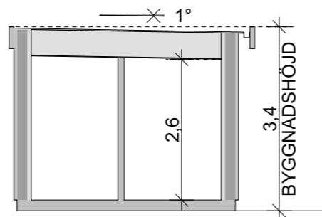
Sektion A1-A1 1:100
