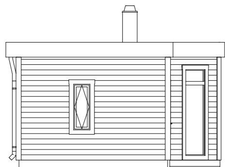
FASAD A1 1:100
