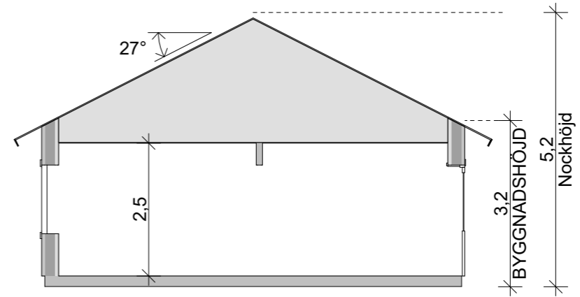
Sektion A 1:100
