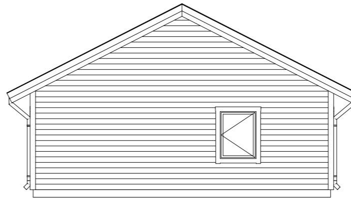
Fasad A2 1:100
