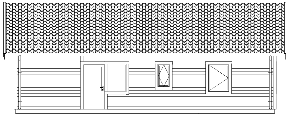
Fasad A1 1:100
