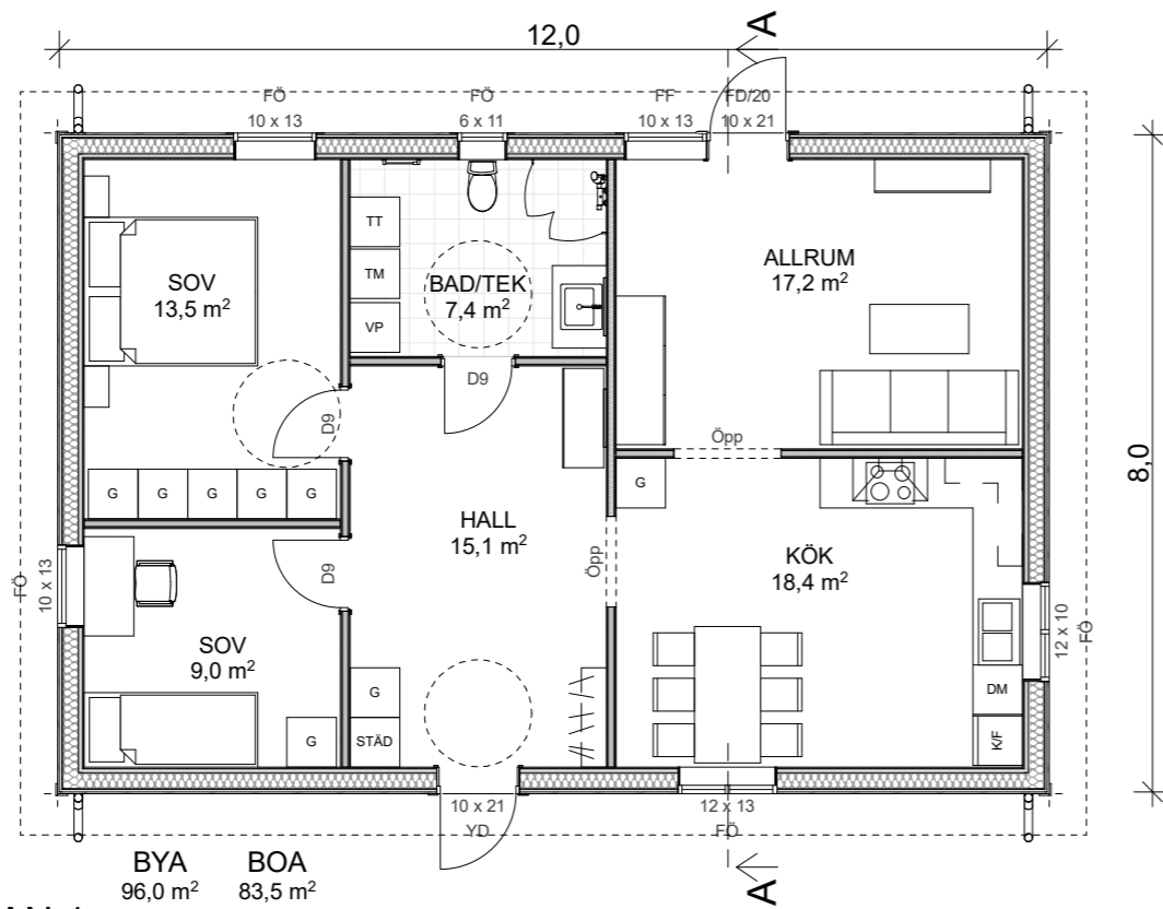
PLAN 1 1:100
